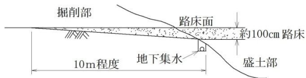
(a) 掘削部路床に置き換えのないとき
