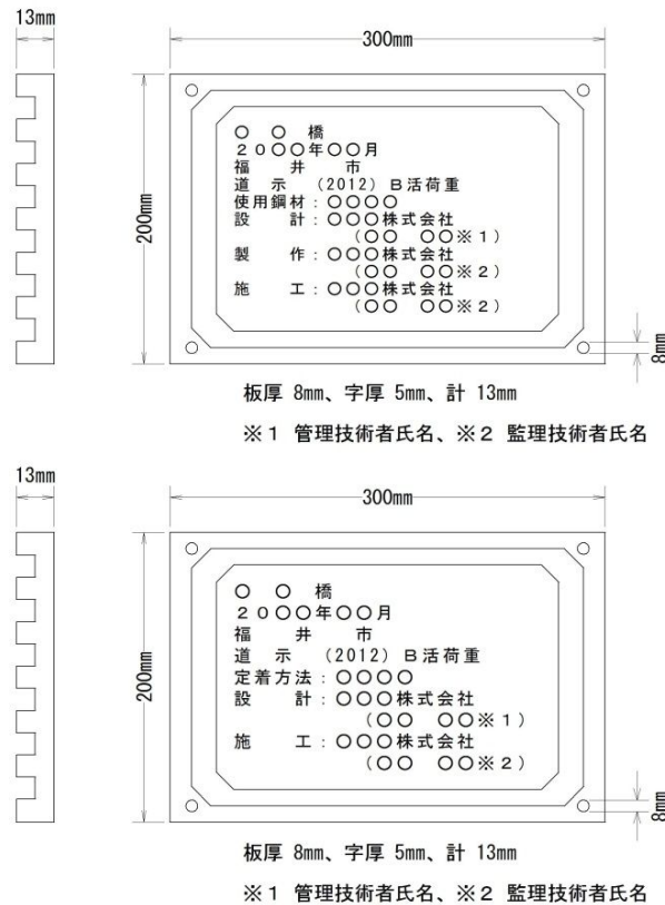
図3 - 2 - 2 - 1 銘板の寸法および記載事項
