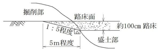
(c) 現地盤がすりつけ区間を長くとることが不経済となる場合
