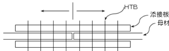
図 3 - 2 - 1 ボルト締付け順序
