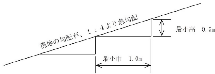
図1-2-1 盛土基礎地盤の段切
