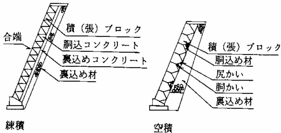
図 3-3 コンクリートブロック工
