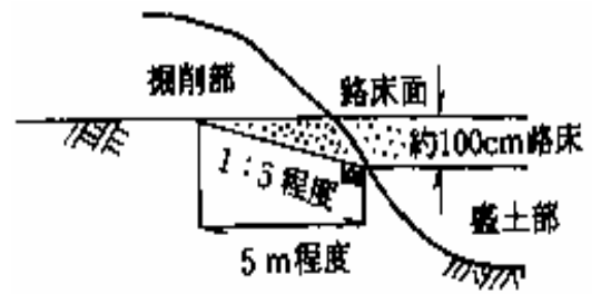
(c) 現地盤が岩ですりつけ区間を長く取ることが不経済となる場合
