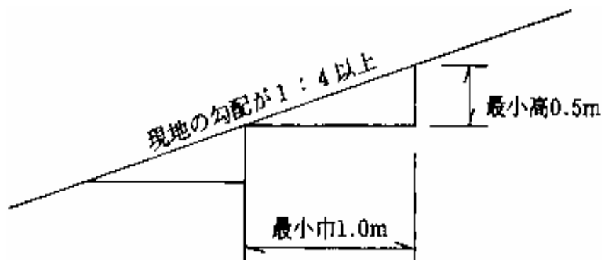
図4-1 盛土基礎地盤の段切
