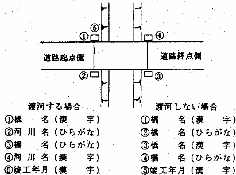
図 5 - 4 橋名板の位置
