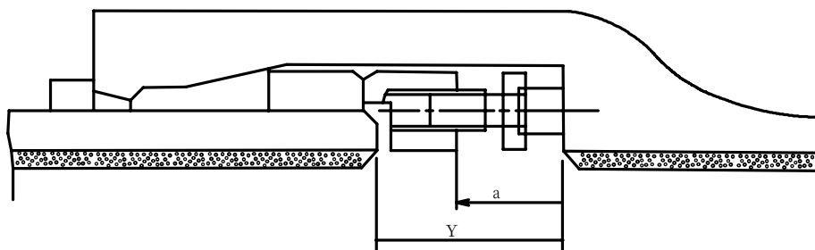
胴付間隔及び締め付け完了時の押輪と受口底部の間隔
