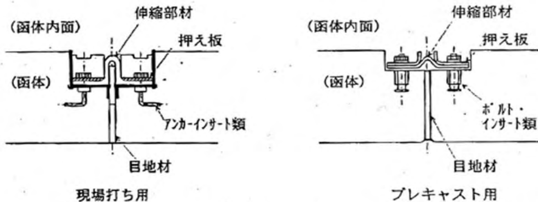
図 3-1 止水板の構造
