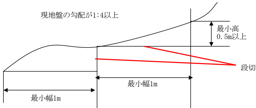
図3-1 盛土基礎地盤の段切
