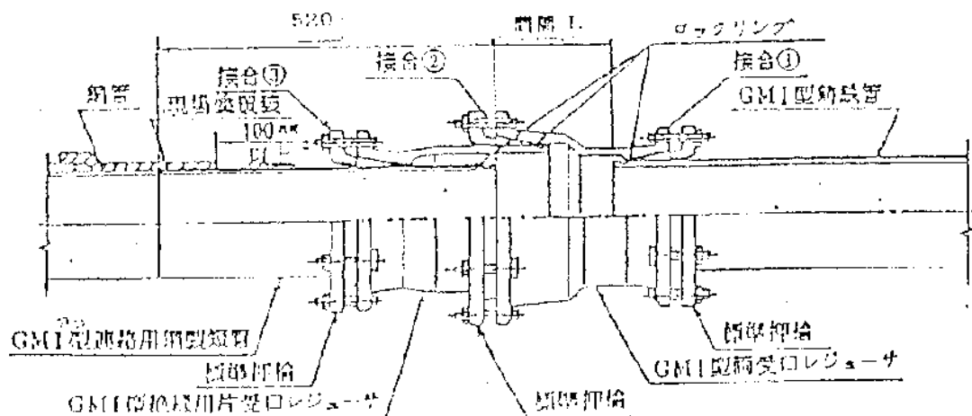
図 5-5 铸铁管及び鋼管の標準接合
