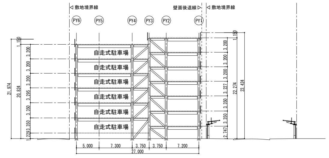
E-E' 断面図
