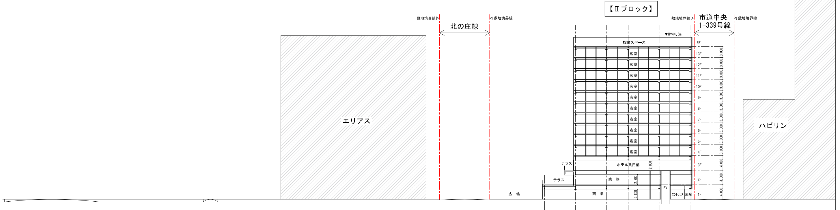
A-A' 断面図
