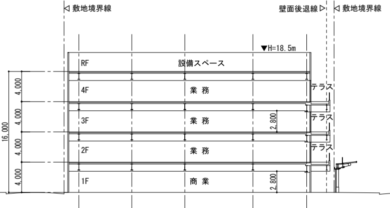
断面図キープラン
