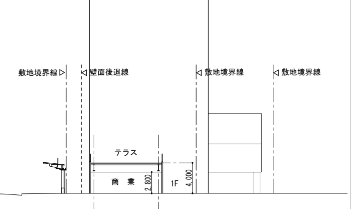
D-D' 断面図
