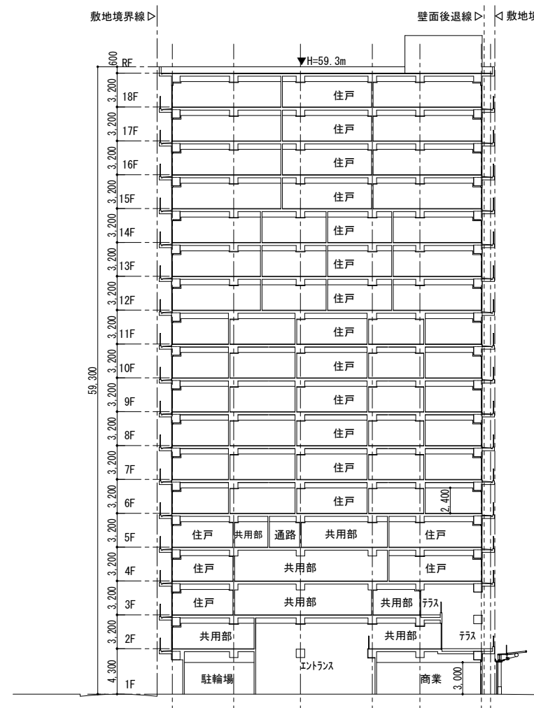
F-F' 断面図
