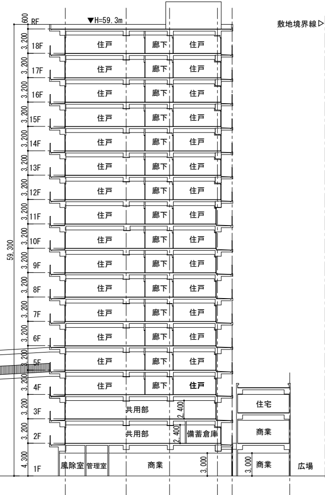
A-A' 断面図
