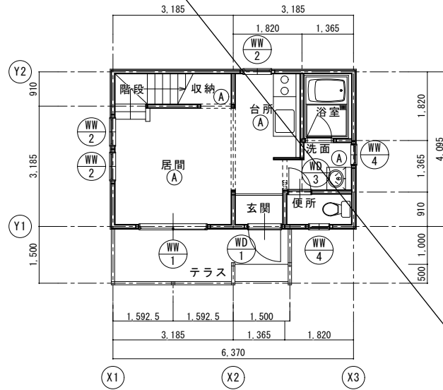
1階平面図 1/100
