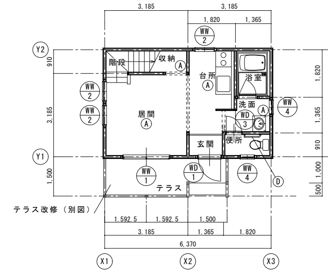
1階平面図 1/100
