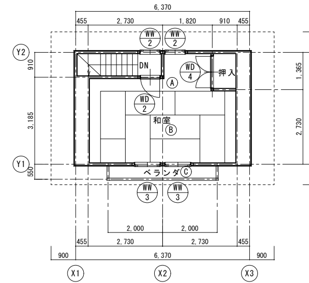
2階平面図 1/100
