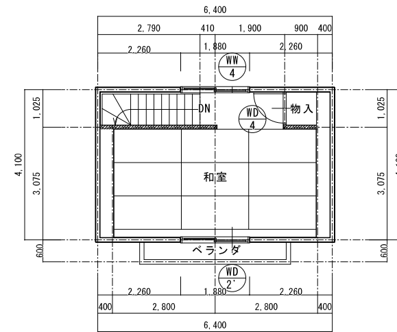
2階平面図 1/100
