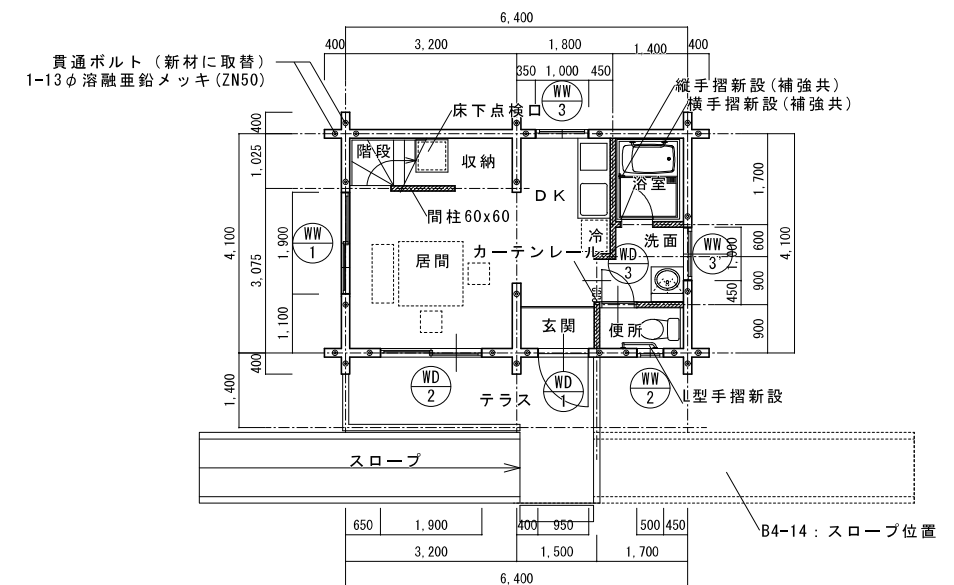
1階平面図 1/100
