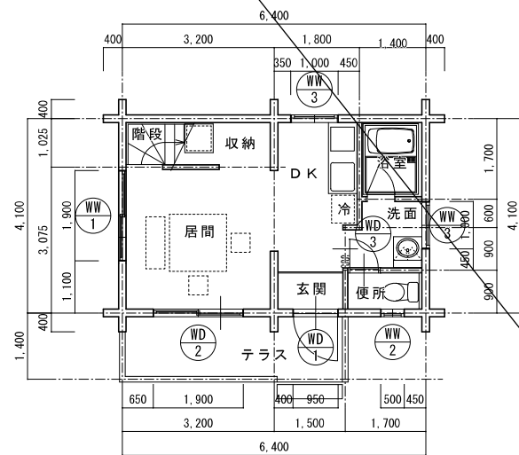
1階平面図 1/100
