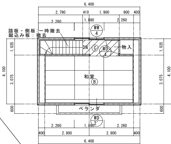
2階平面図 1/100
