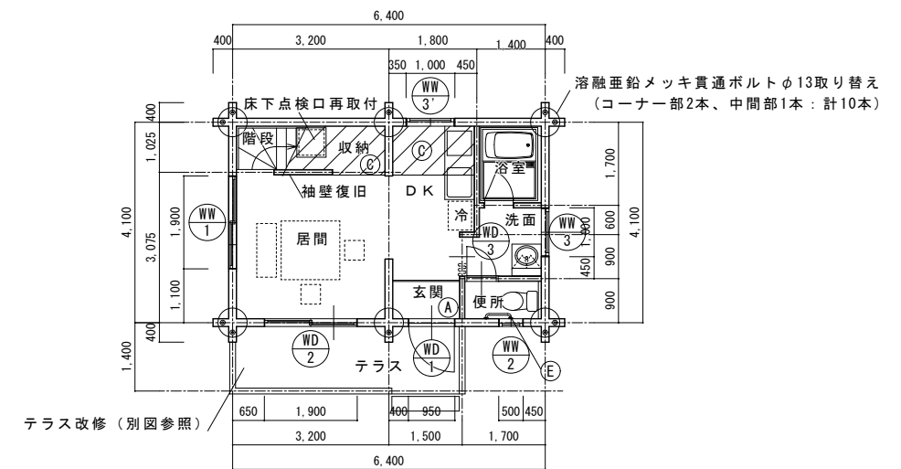
1階平面図 1/100
