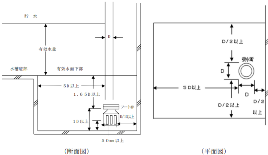
図2-1 (地下又は床下水槽を用いサクシオンピットを設ける場合)
