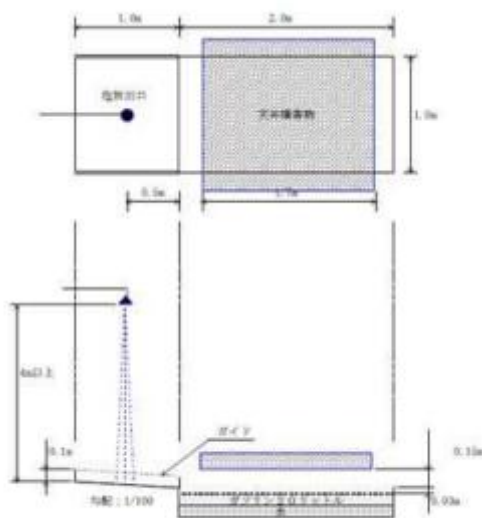
図2 下方放出方式
