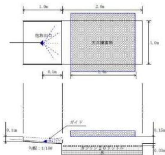
図1 水平放出方式
