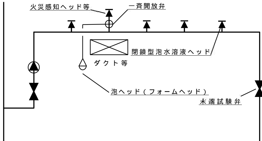
第5図【一斉開放弁泡ヘッド併用型平面式泡消火設備の構成例】
