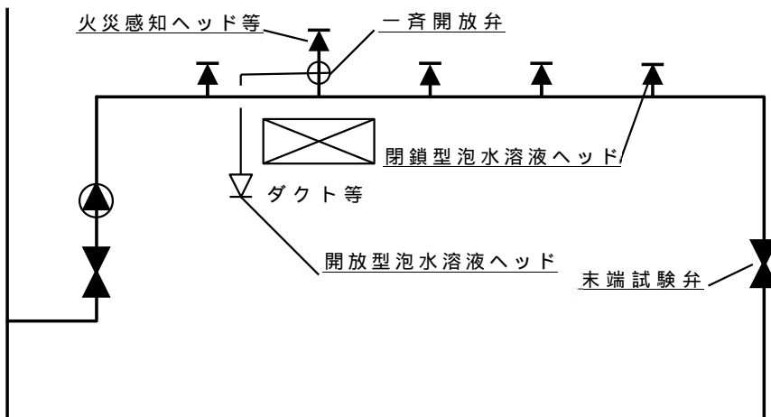
第4図【一斉開放弁開放ヘッド併用型平面式泡消火設備の構成例】
