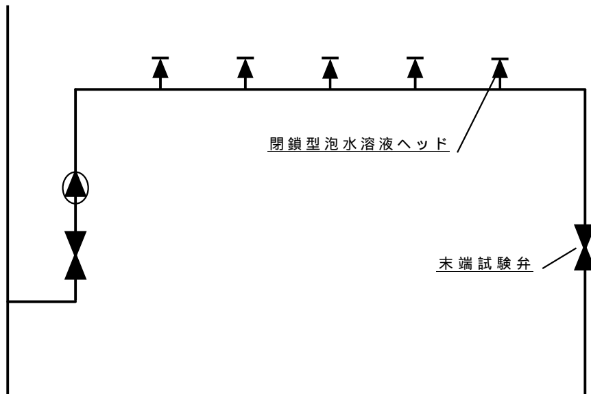
第1図【単純型平面式泡消火設備の構成例】
