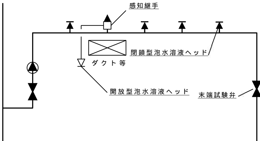
第2図【感知継手開放ヘッド併用型平面式泡消火設備の構成例】
