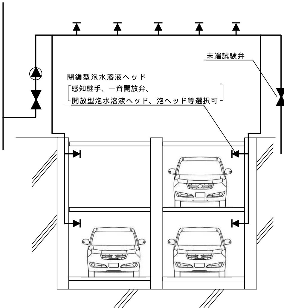
第6図【機械式泡消火設備の構成例】
