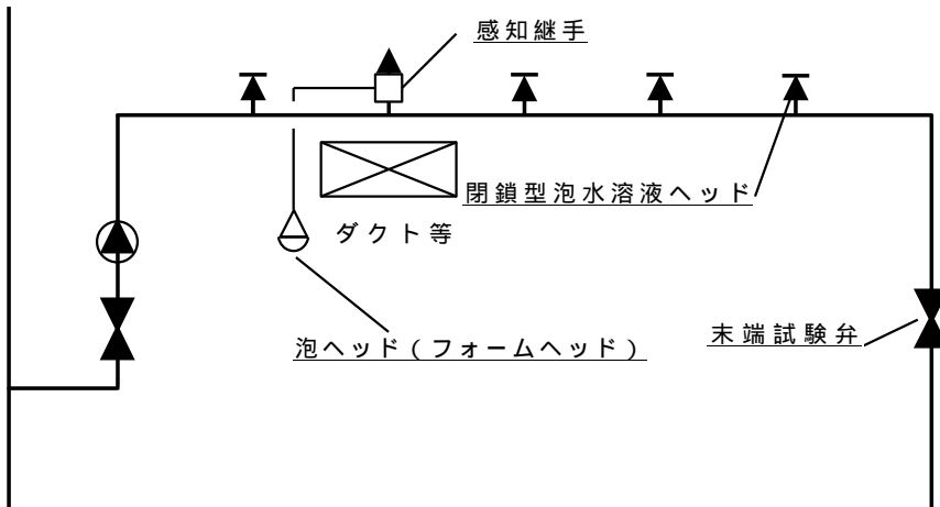
第3図【感知継手泡ヘッド併用型平面式泡消火設備の構成例】
