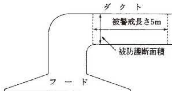
第4図【ダクトの被警戒長さ及び被防護断面積】
