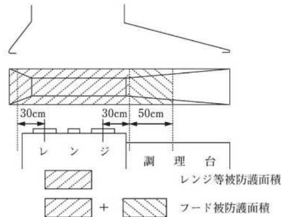
第2図【レンジ又はフライヤーの被防護面積よりフードが大きい場合のフード被防護面積例】
