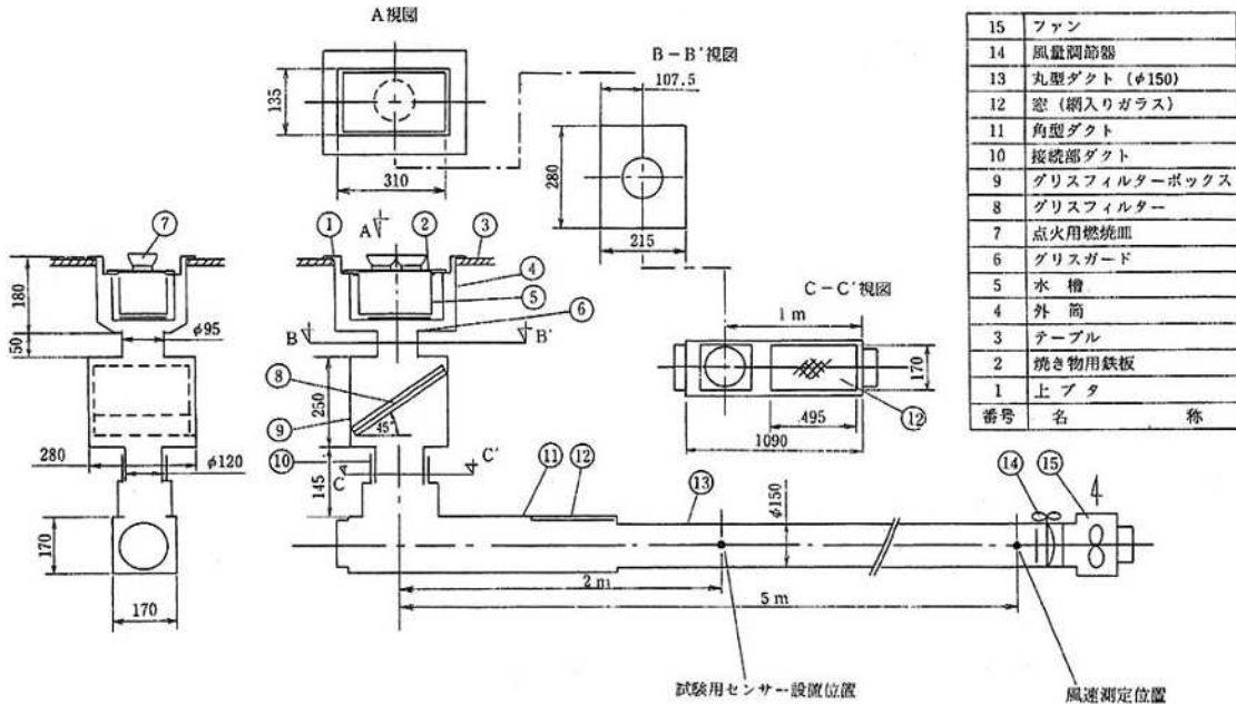
別図2【消火試験図】
