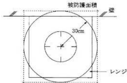
第5図【レンジの被防護面積(コンロが1口の場合の例)】
