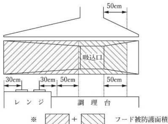
第3図【ダクト吸込口がレンジの直上部以外の位置にある場合のフードの被防護面積の例】
