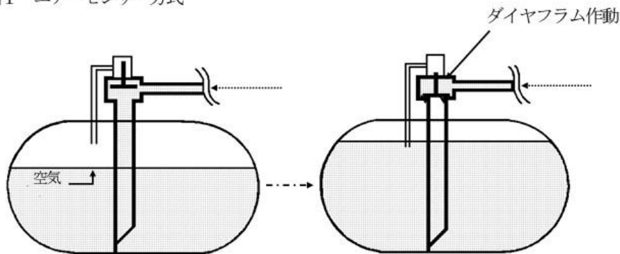
例図1 エアーセンサー方式
