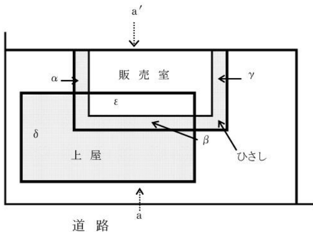
ア 平面図
