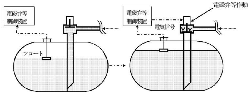
例図3 液面計連動型遮断方式
