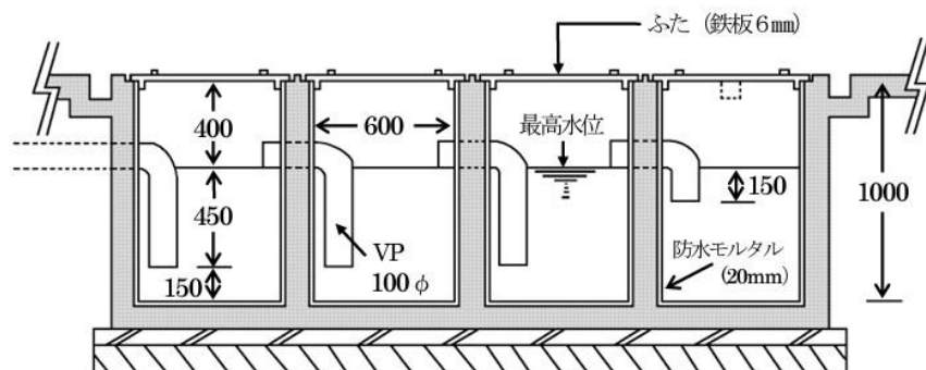
断面図
