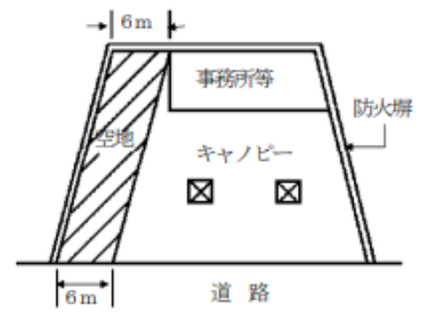
(4) 空地进行斜めに取る場合
