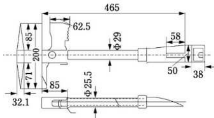
図4【破壊器具】
