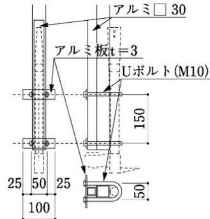
図5【固定方法】
