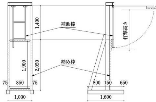
図1【本体】
