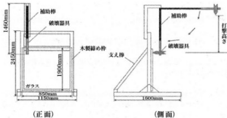
図 1 【本体】
