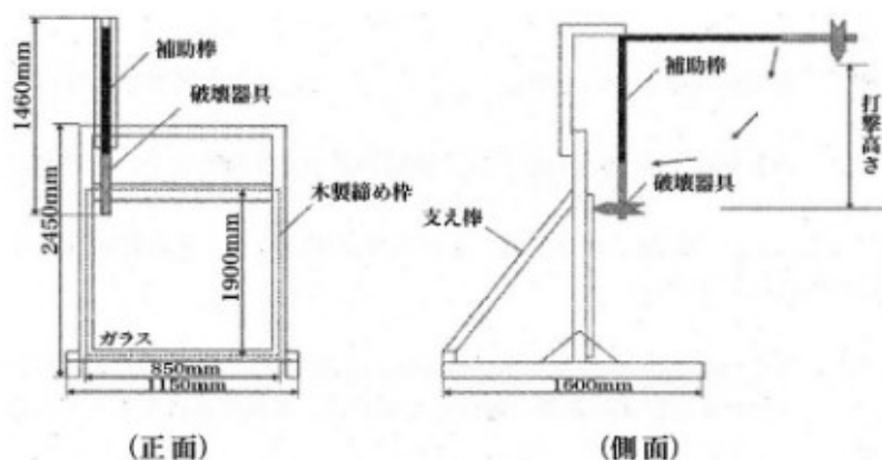
図 1【本体】
