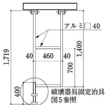
図3【補助棒】
