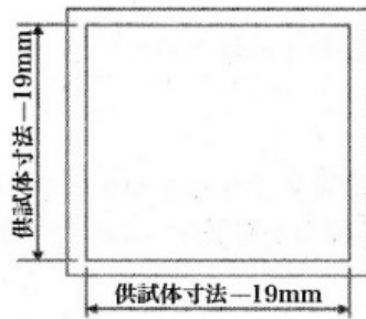
第2【締め枠】
