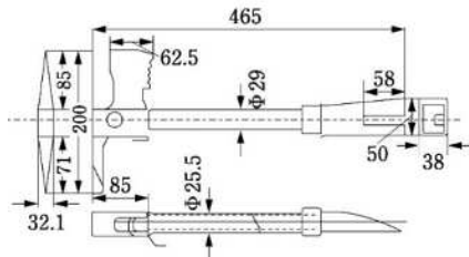
図4【破壊器具】
