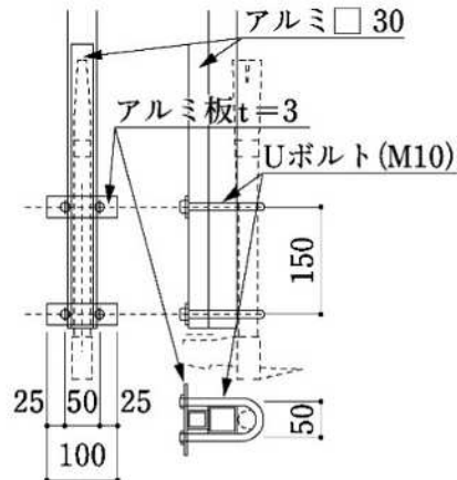
図5【固定方法】
