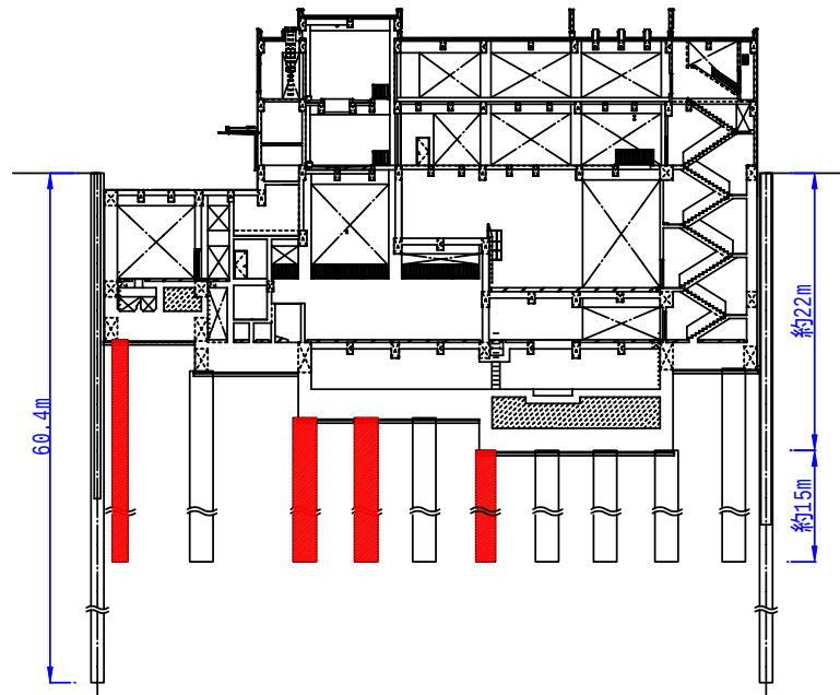
断面図
