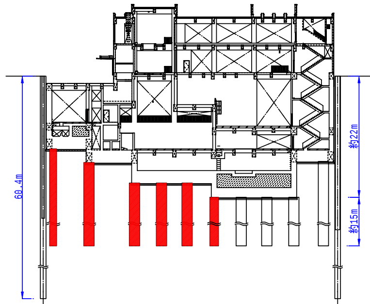
断面図
