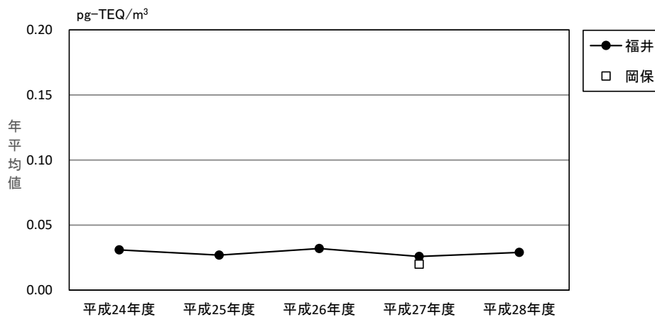
図 4.1-12 ダイオキシン類の経年変化(平成24年度～平成28年度)
