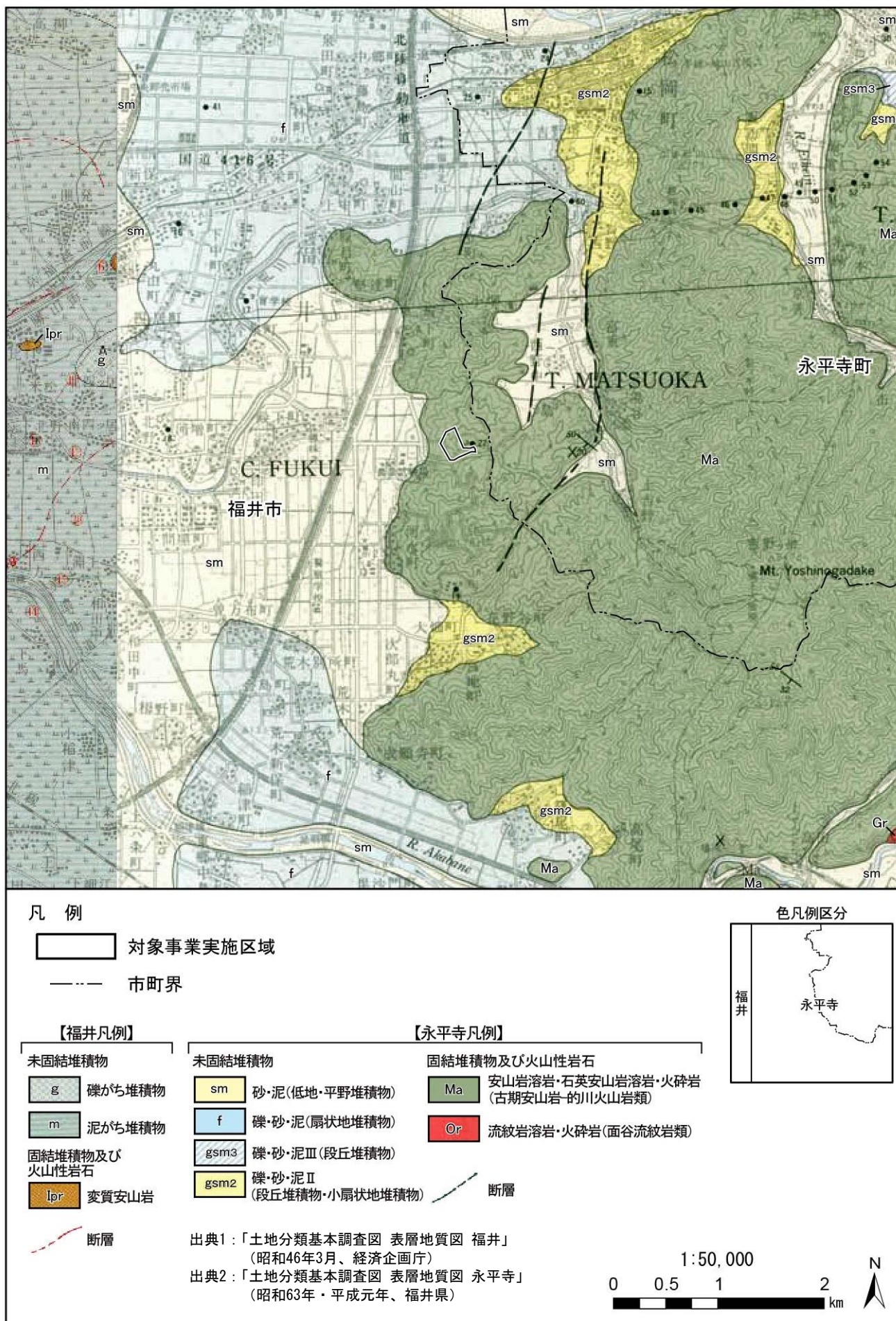
図 4.1-19 表層地質図
