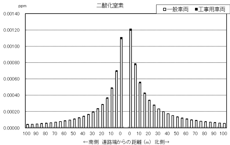
図 8.1-18(1) 工事用車両の運行に伴う二酸化窒素の予測結果 (年平均値)
