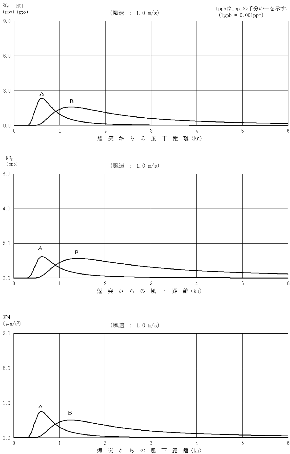
図 8.1-21 煙突排ガスによる一般的な気象条件時の寄与濃度予測結果 (1時間値、最大着地濃度出現時)
