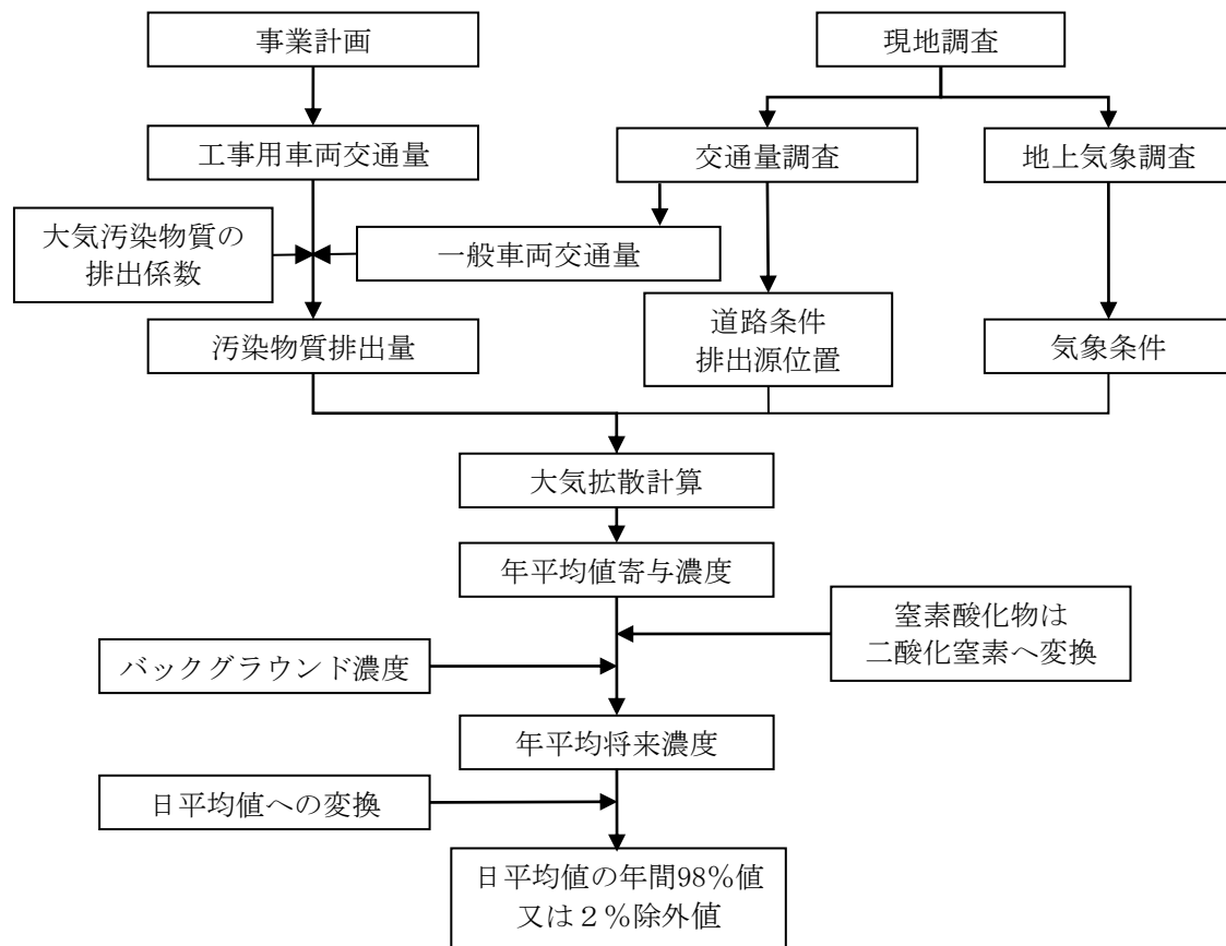
図 8.1-16 工事用車両の運行に伴う二酸化窒素・浮遊粒子状物質の予測手順
