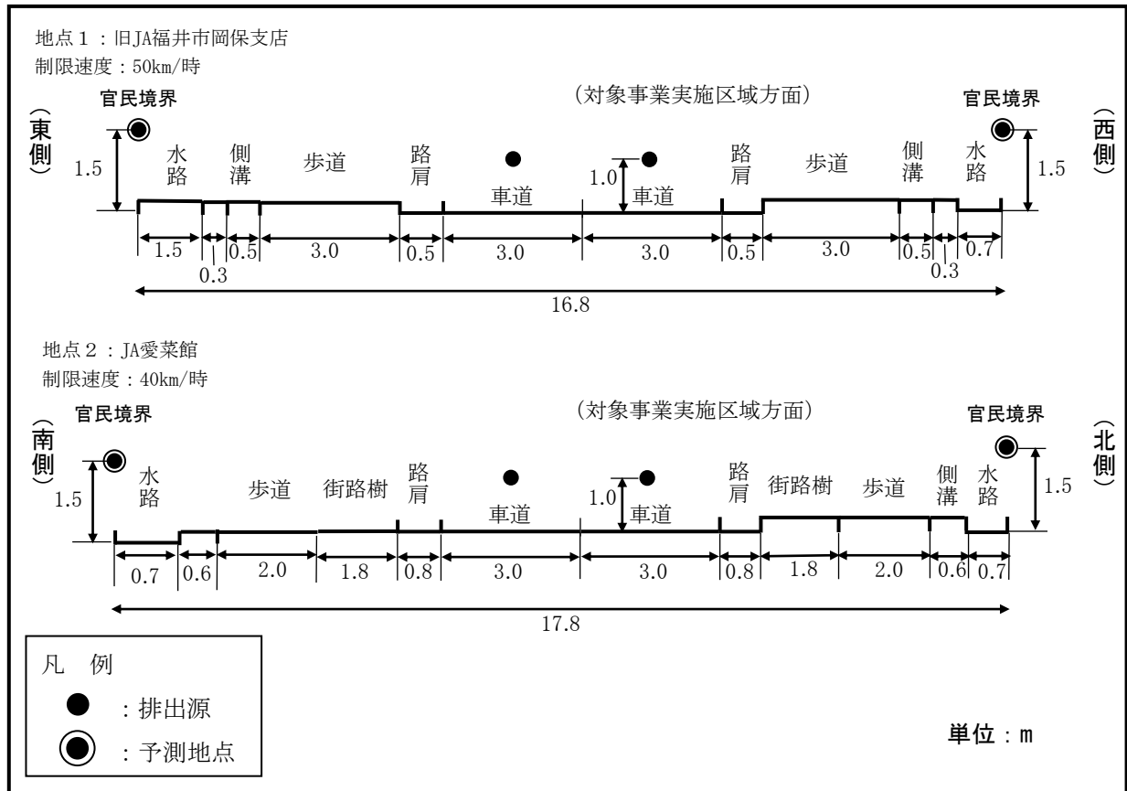
図 8.1-10 工事用車両の運行に伴う大気質の予測地点の断面構成
