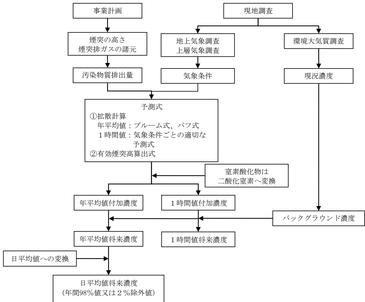
図 8.1-19 施設の稼働による大気質の予測
