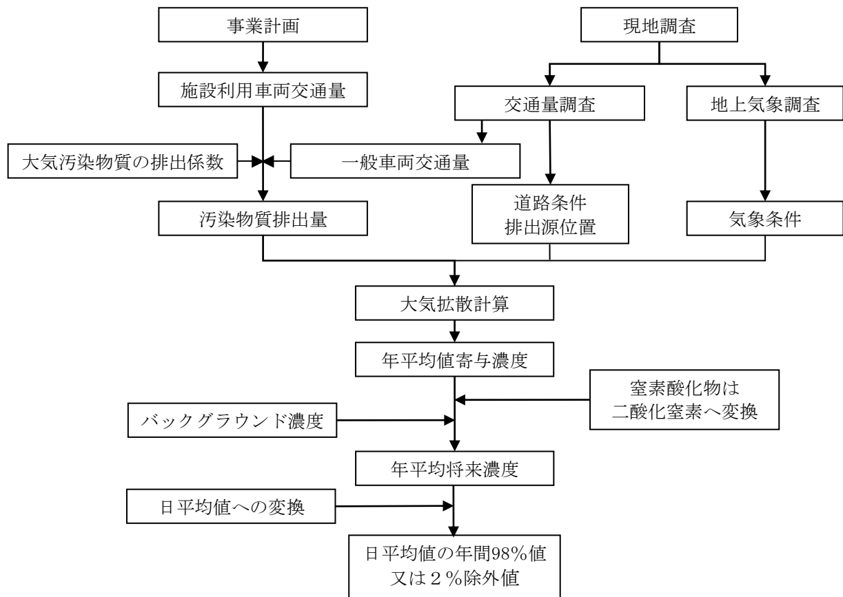
図 8.1-25 施設利用車両の走行による大気質の予測手順
