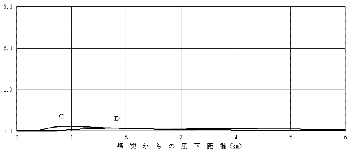
図 8.1-23 煙突排ガスによるダウンウォッシュ時の寄与濃度予測結果 (1時間値、最大着地濃度出現時)
