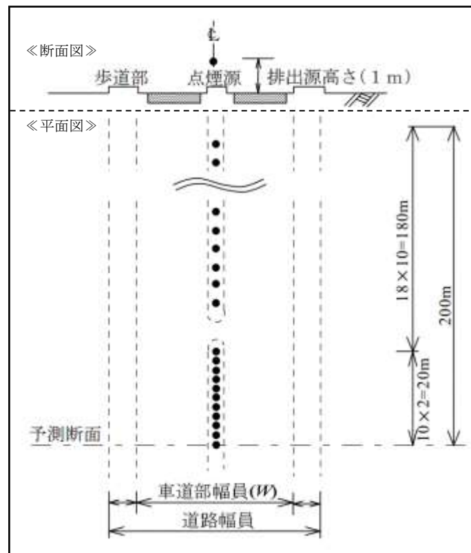
図 8.1-17 煙源の位置
