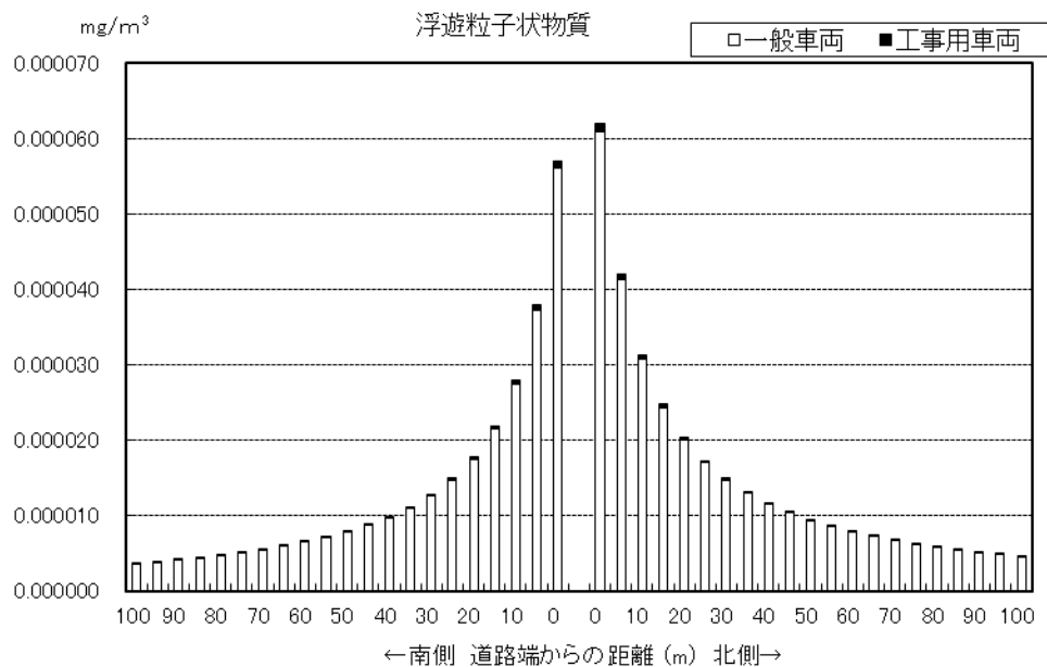
図 8.1-18(2) 工事用車両の運行に伴う浮遊粒子状物質の予測結果 (年平均値)
