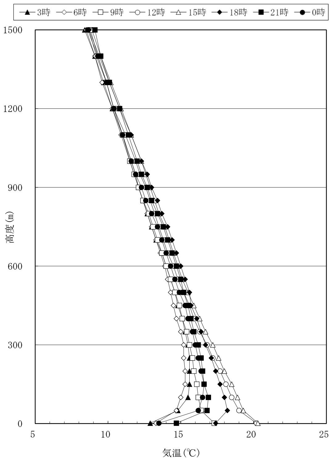
図 8.1-4 鉛直気温調査結果（通年）
