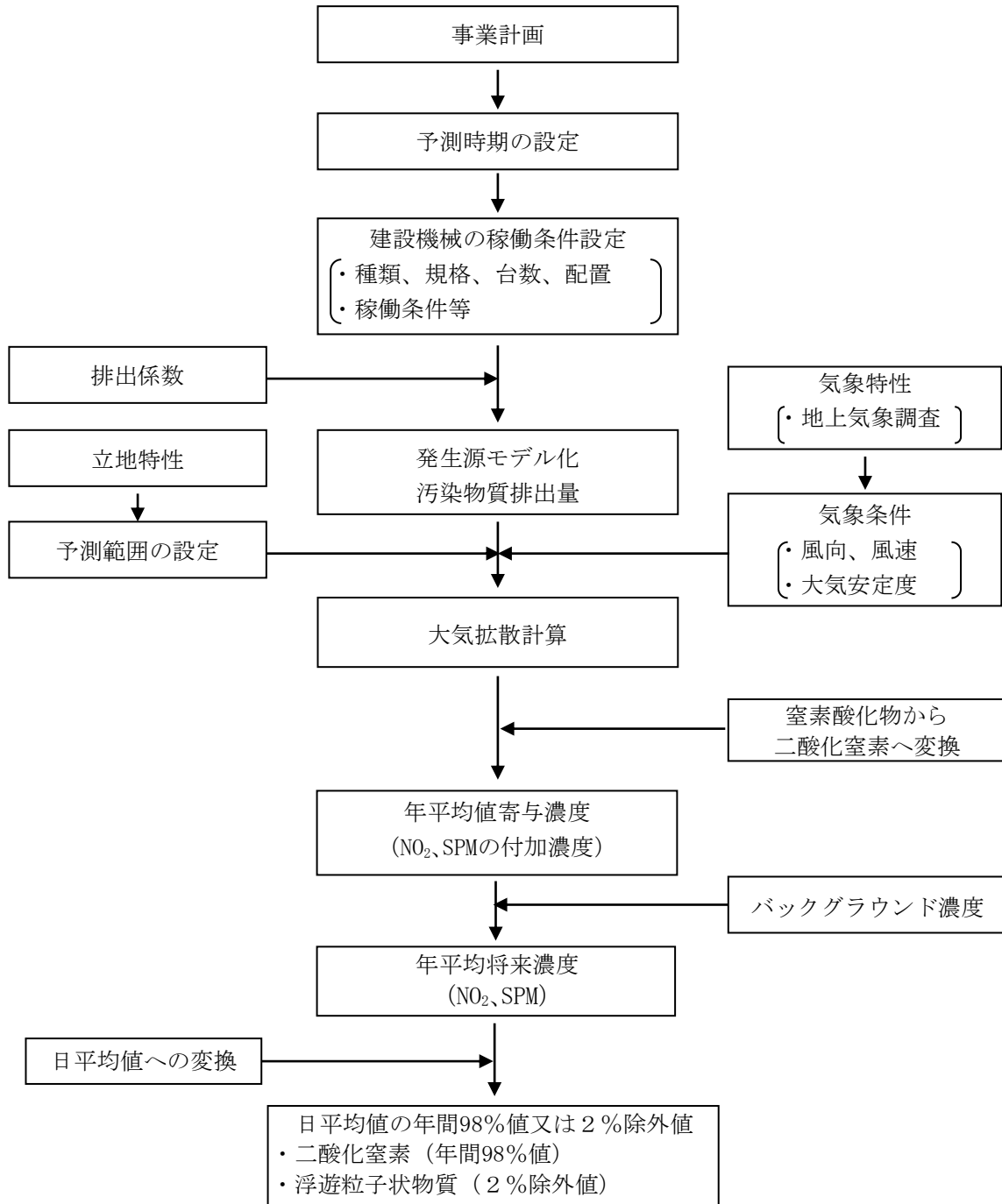
図 8.1-13 建設機械の稼働による大気質の予測手順
