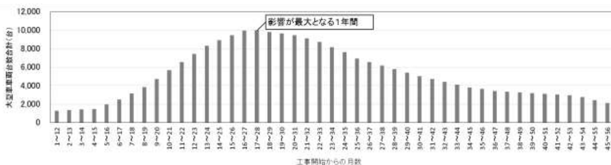
図 8.1-15 工事用車両の運行に伴う二酸化窒素・浮遊粒子状物質の予測対象時期
