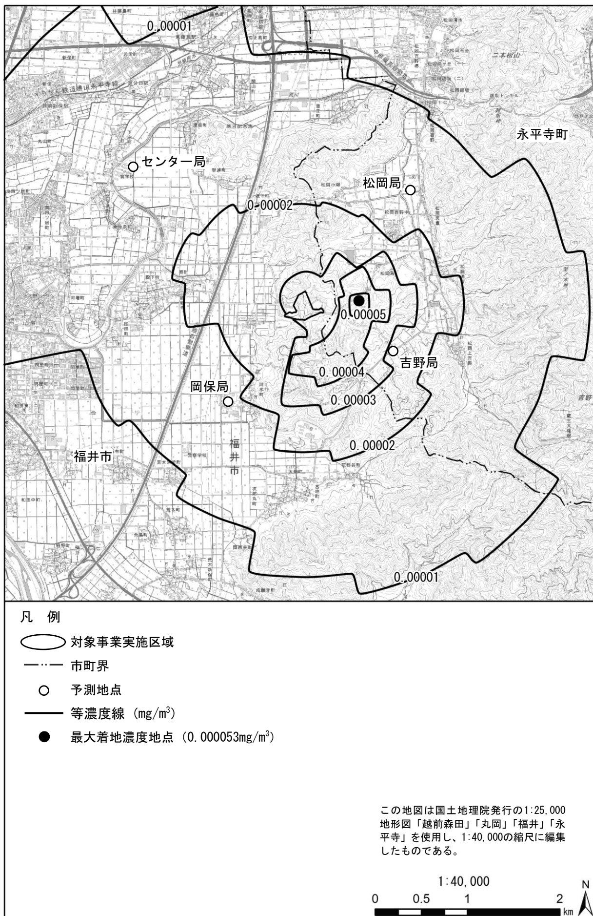
図 8.1-20(3) 煙突排ガスによる浮遊粒子状物質濃度予測結果（年平均値）
