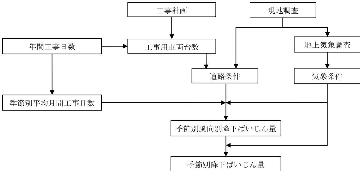
図 8.1-9 工事用車両の運行に伴う粉じんの予測手順
