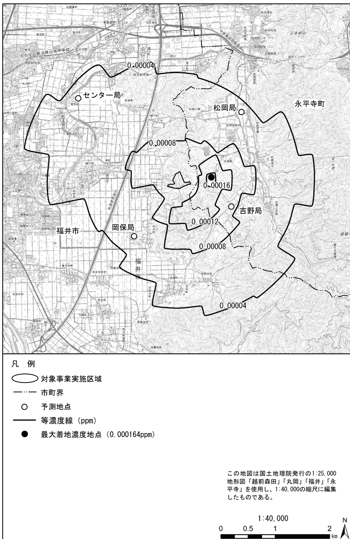
図 8.1-20(1) 煙突排ガスによる二酸化硫黄濃度予測結果 (年平均値)
