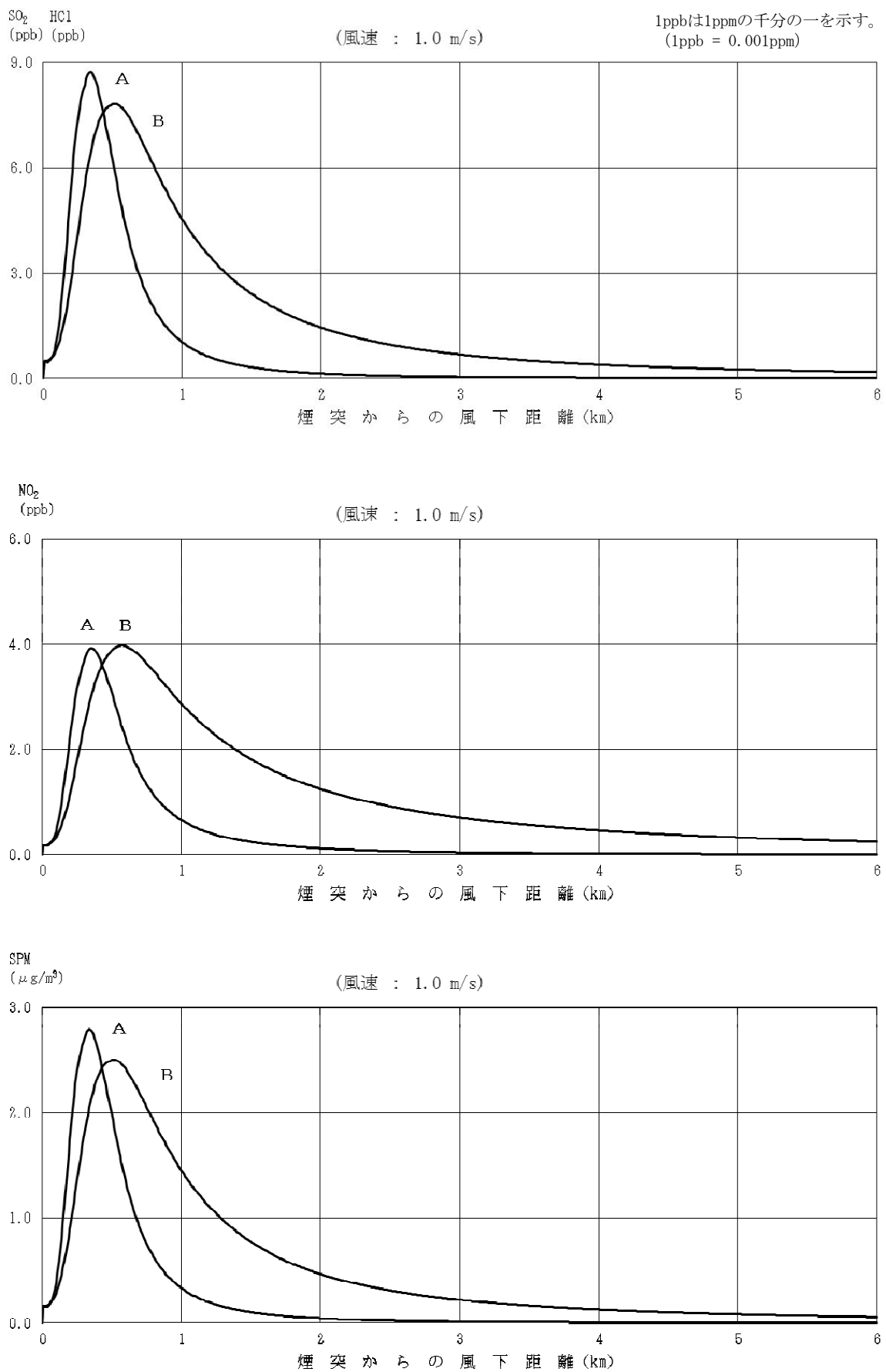
図 8.1-24 煙突排ガスによるダウンドラフト時の寄与濃度予測結果 (1 時間値、最大着地濃度出現時)
