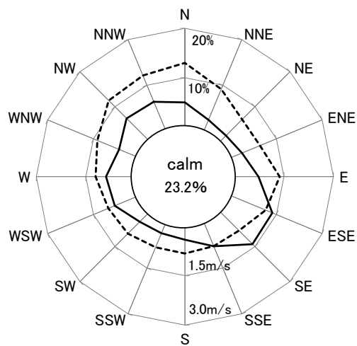
図 8.1-3 風配図
