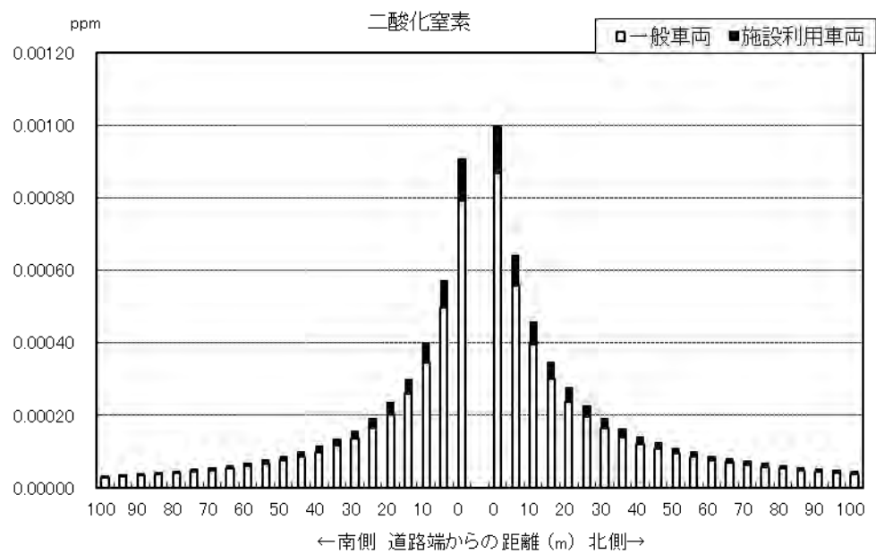
図 8.1-26(1) 施設利用車両の運行に伴う二酸化窒素の予測結果 (年平均値)
