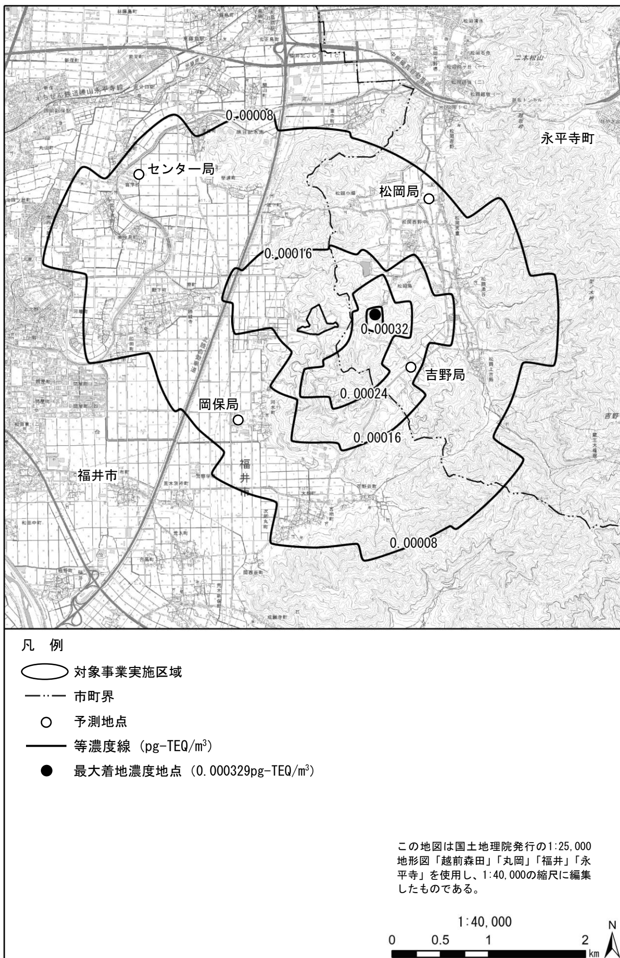
図 8.1-20(4) 煙突排ガスによるダイオキシン類濃度予測結果 (年平均値)
