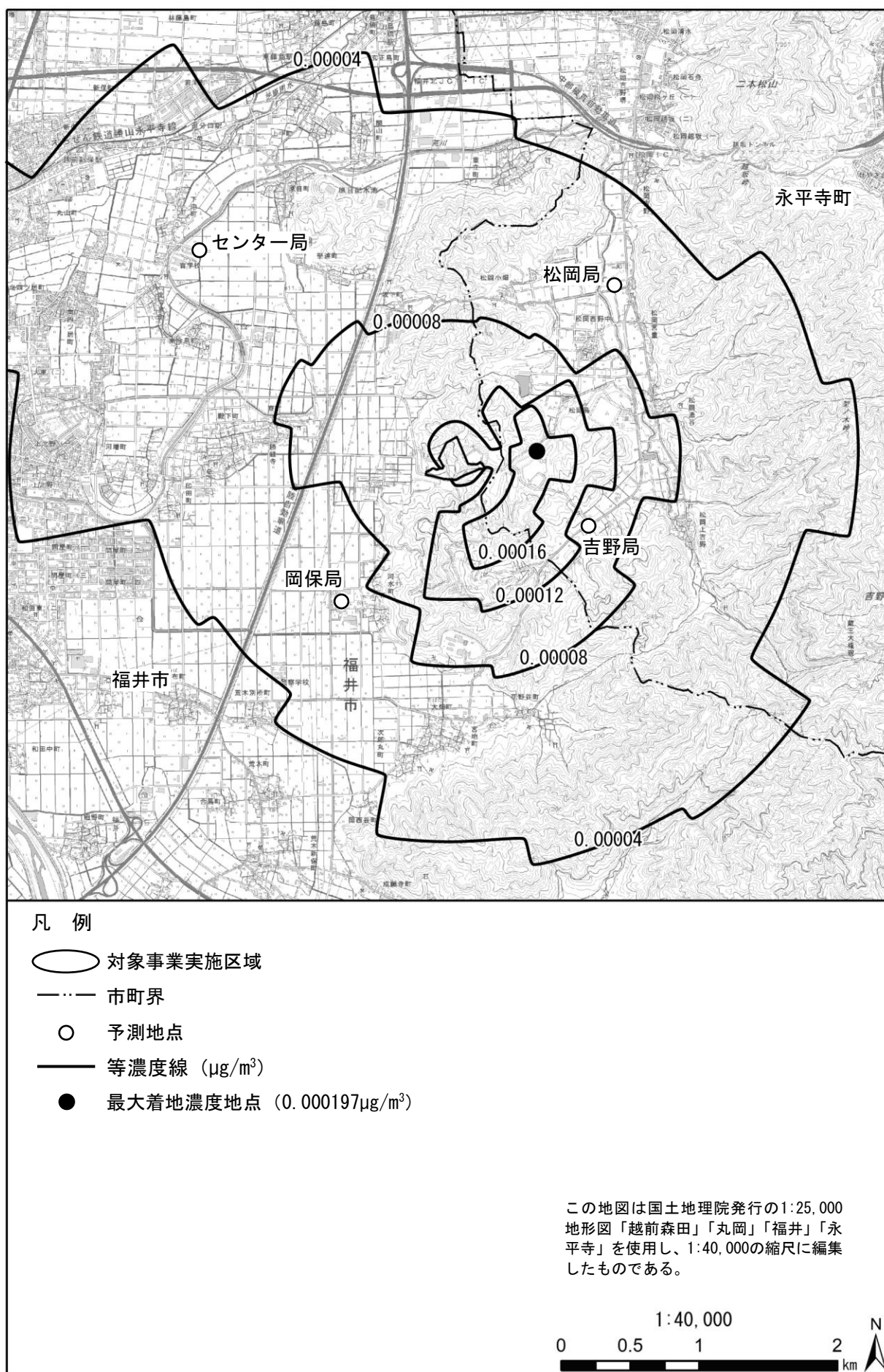
図 8.1-20(5) 煙突排ガスによる水銀濃度予測結果（年平均値）
