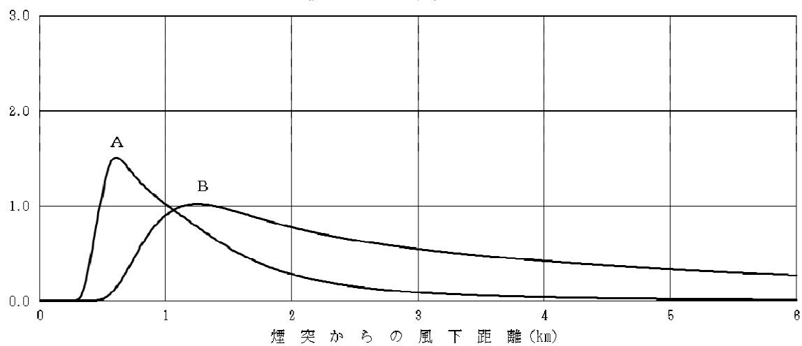
図 8.1-22 煙突排ガスによる上層逆転発生時の寄与濃度予測結果 (1時間値、最大着地濃度出現時)
