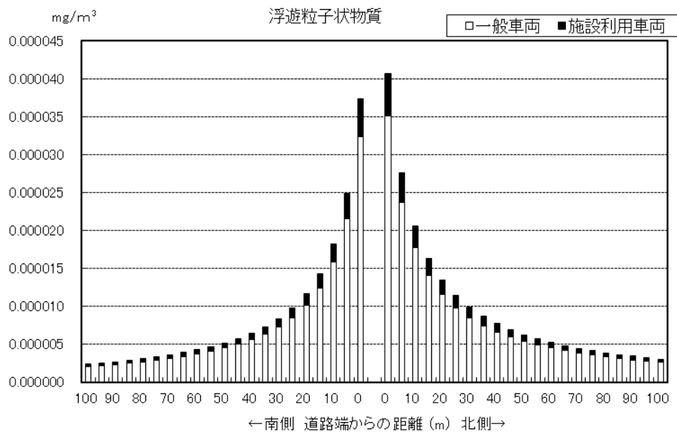
図 8.1-26 (2) 施設利用車両の運行に伴う浮遊粒子状物質の予測結果 (年平均値)
