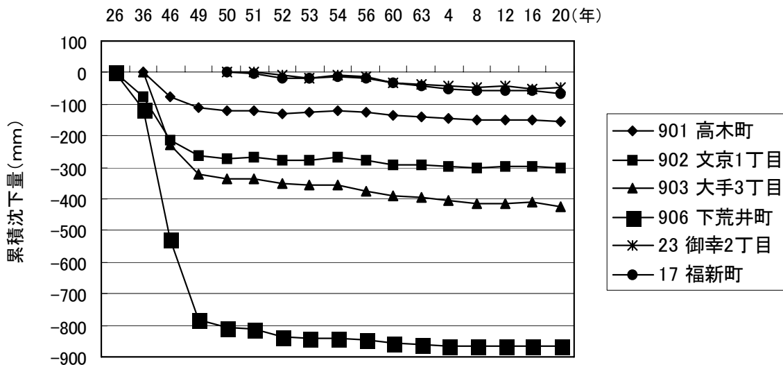
水準点の経年変化
