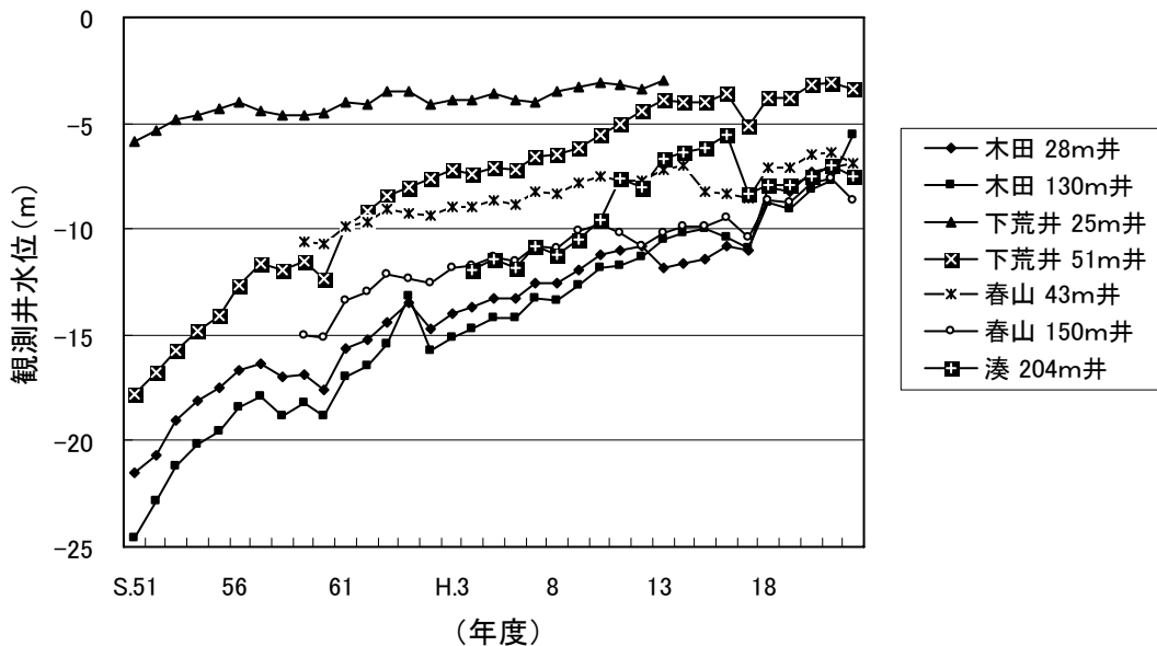
地下水 (経年変化)
