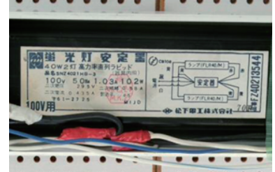
③ 安定器の銘板の写真をとり記載内容を確認
