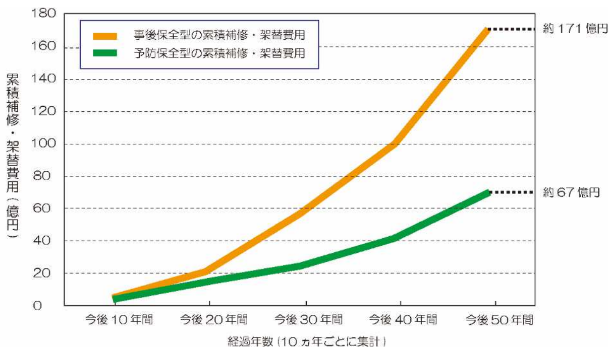
図3 補修コスト比較グラフ
