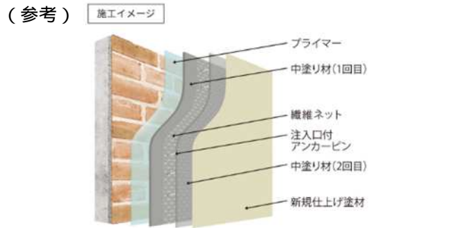
【体育館：透明樹脂系タイル張り仕上げ外壁複合改修工法】
