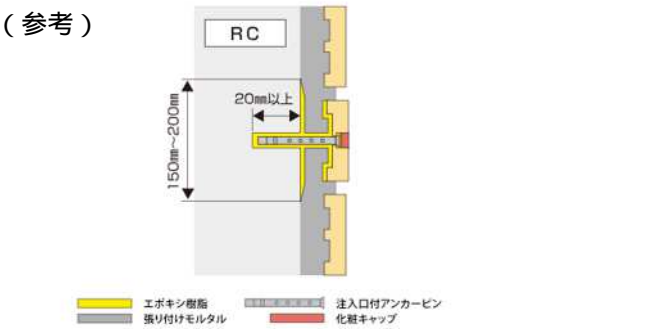
【校舎：注入口付アンカーピンニングエポキシ樹脂注入タイル固定工法】
