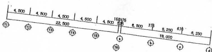
本館B棟・体育館 R階平面図 S=1/300
