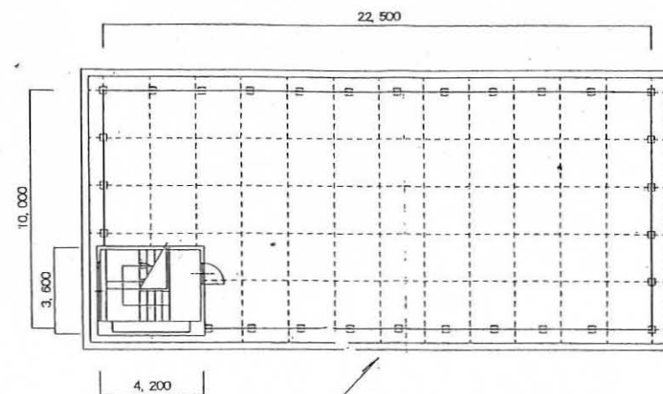
別館 3階平面図 S=1/200
