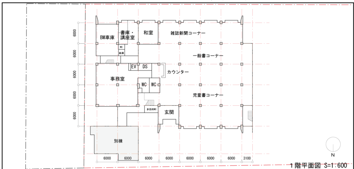
中置書架：柱間隔は 6\text{m} \times 1/3 = 2\text{m} ピッチで余 裕があるものの、裾広がり型のため高書架上 部の資料が取りづらい
