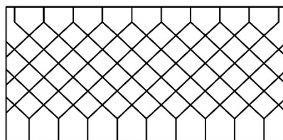
図3-2-4 谷 積
