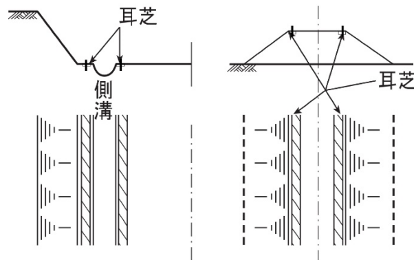
図3-2-6 耳芝
