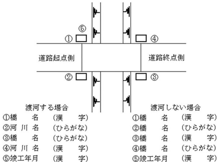
図3-2-2(2) 橋名板の位置
