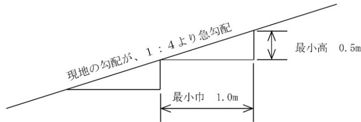
図1-2-1 盛土基礎地盤の段切
