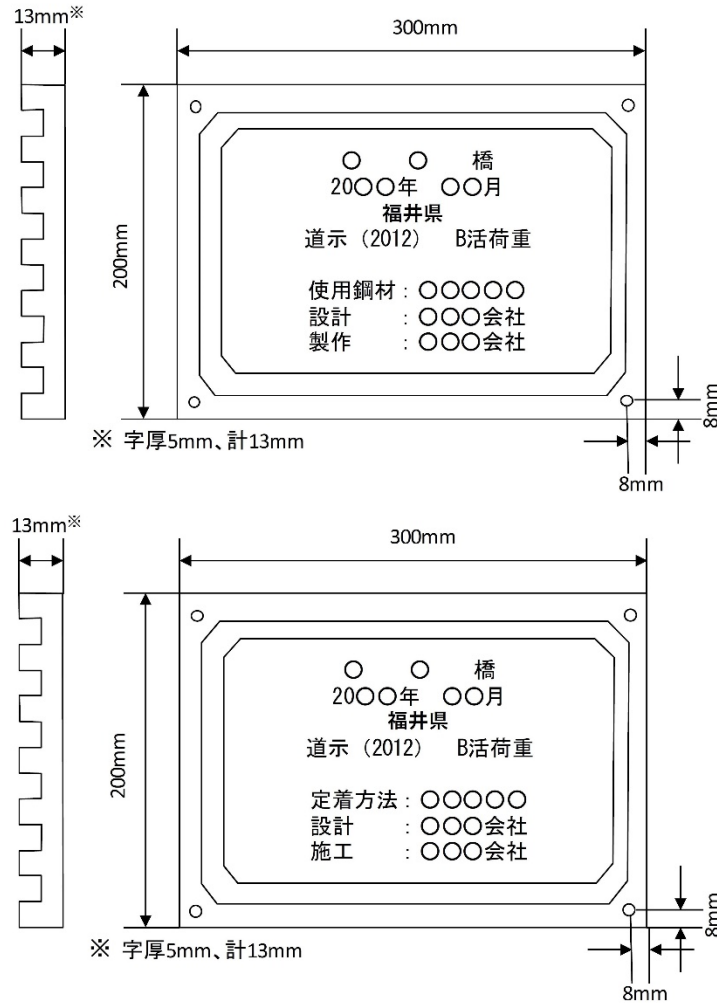
図3-2-2(1) 銘板の寸法および記載事項
