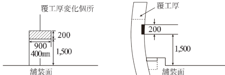
図10-6-1 覆工厚変化箇所の刻示標準図
