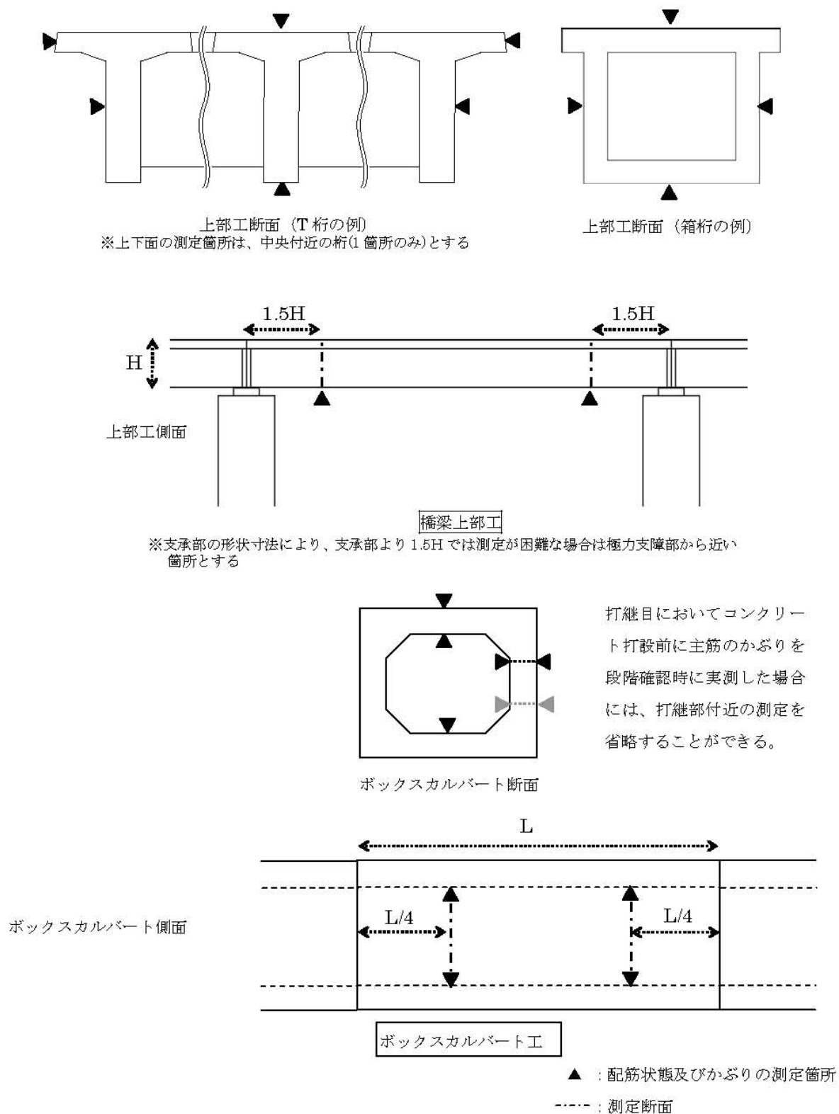
図 2 配筋状態及びかぶりの測定箇所 (例) (その 2)
