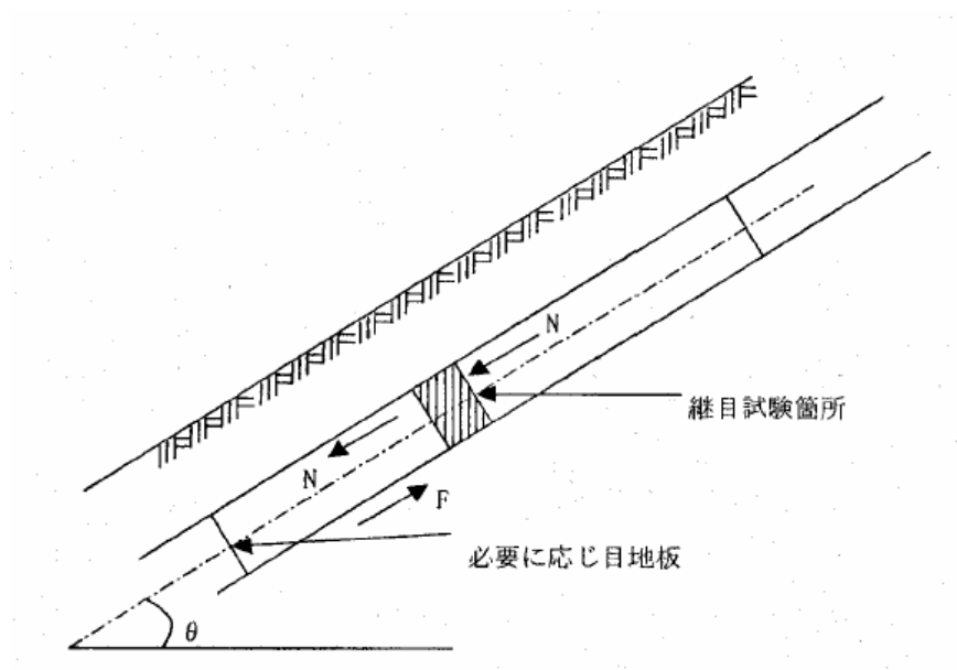
図 2-2 継目試験箇所及び力
