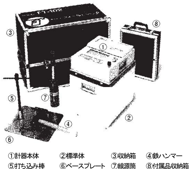
図－4 計器の構成例（透過型）
