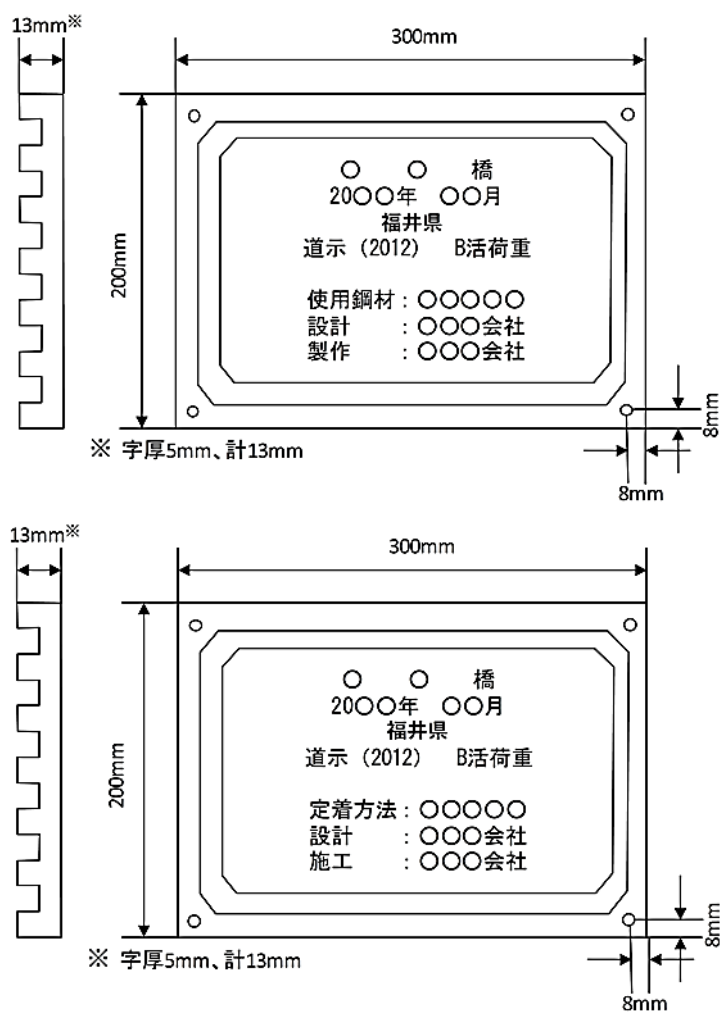
図3-2-2 銘板の寸法および記載事項
