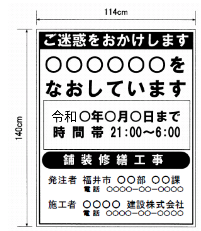
図1-1-2 標示板
