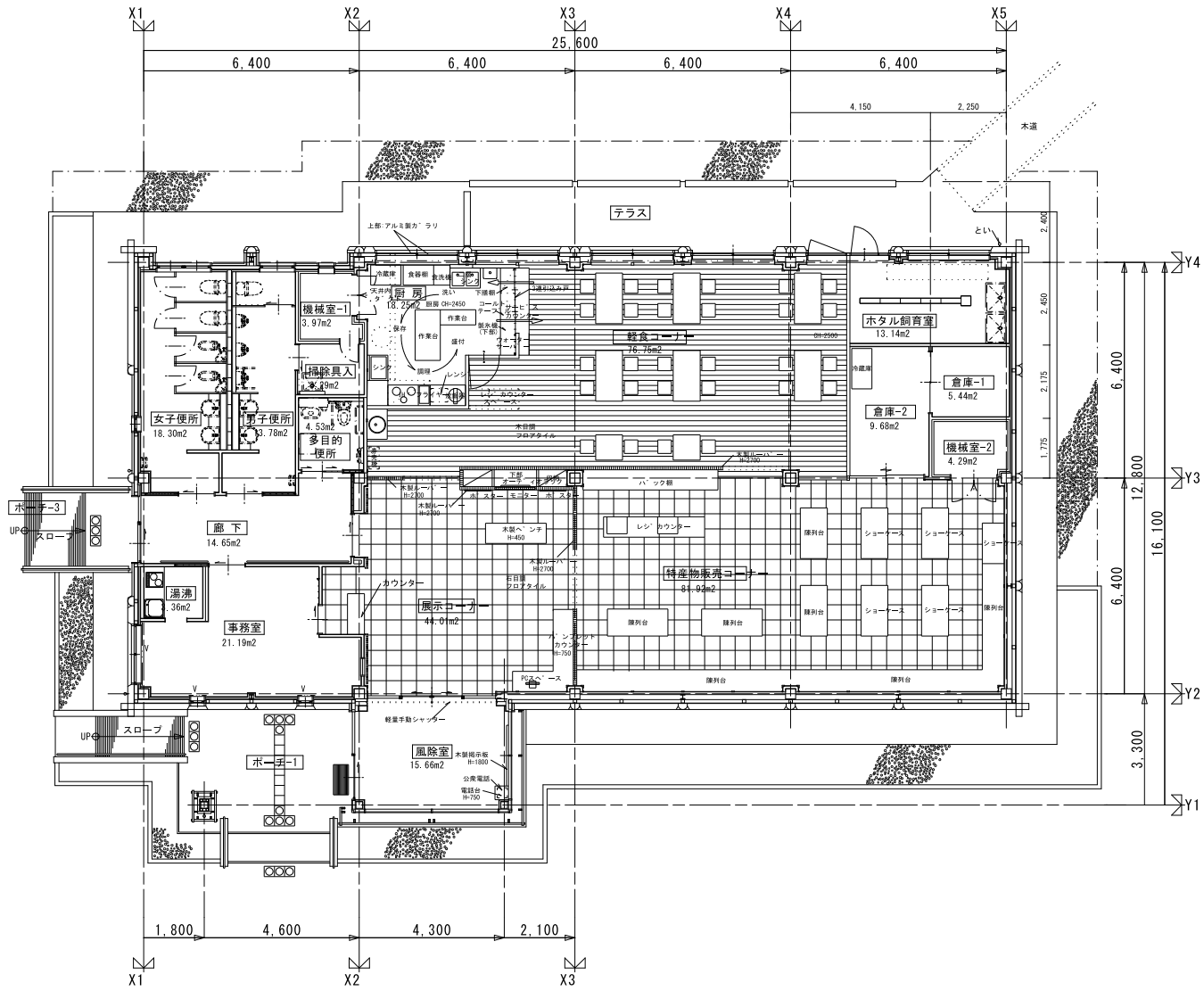
平面図 SCALE 1:100
