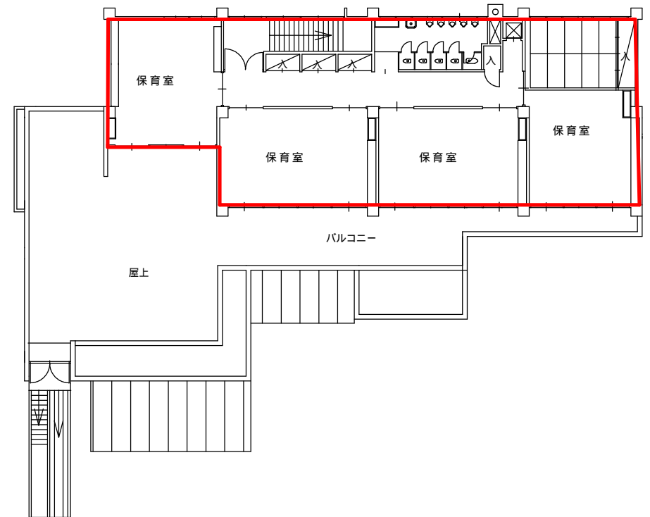
2階平面図
