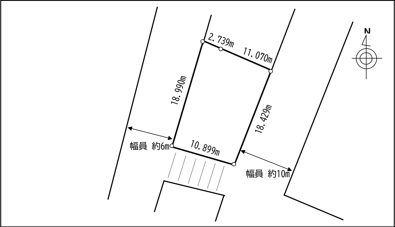
明細図（略図）
