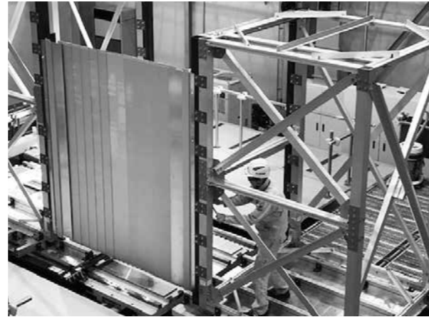
3次元振動台を使って性能を検証しているジョイントカバー（写真左側の金属板）
