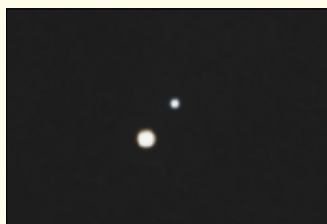
二重星のアルビレオ
